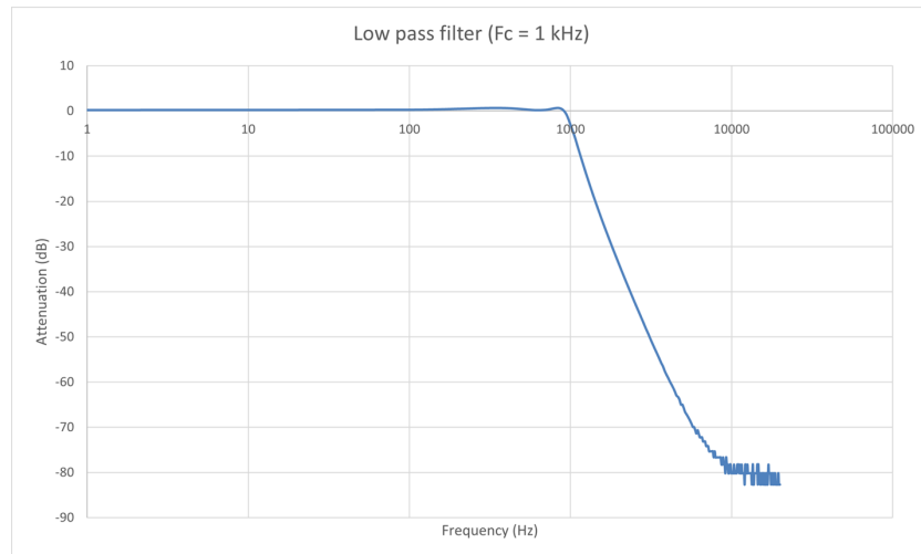
FIGURE 5.9 : Filtre passe-bas Chebyshev : Diagramme de Bode
