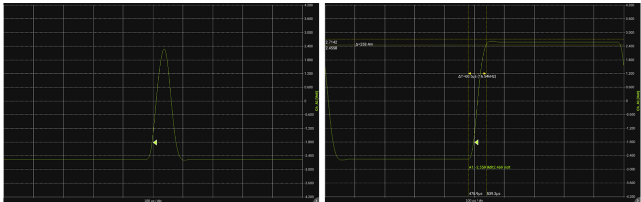
FIGURE 5.12 : Filtre passe-bas Bessel : Réponses impulsionnelle et indicielle
