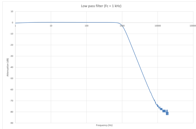
FIGURE 5.7 : Filtre passe-bas Butterworth : Diagramme de Bode
