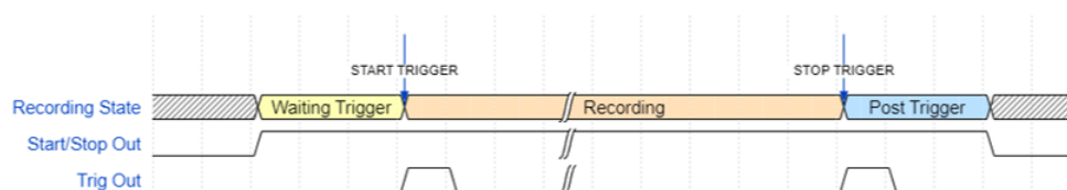
FIGURE 3.36 : Chronogramme Déclencheur
