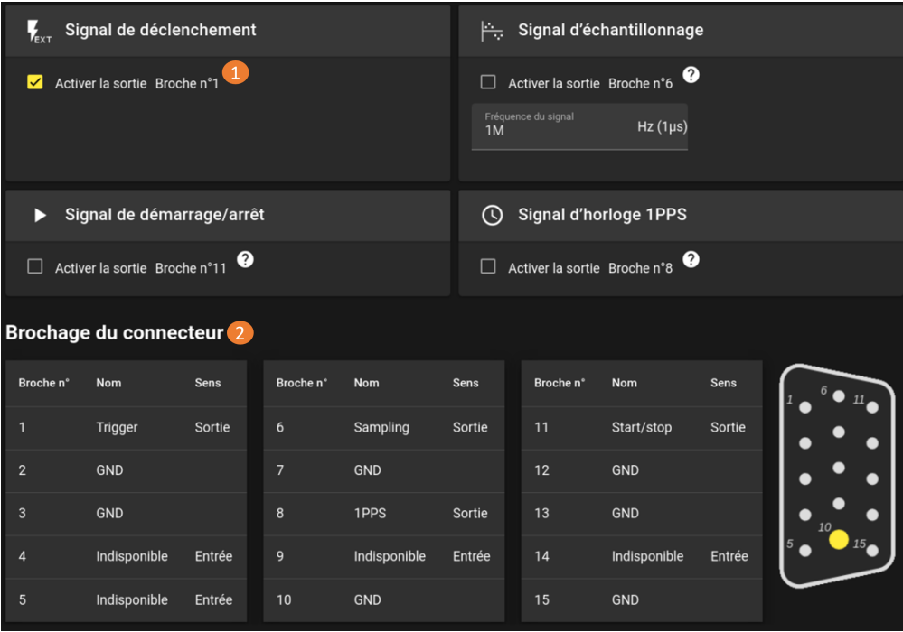
FIGURE 3.34 : Menu Synchro externe
