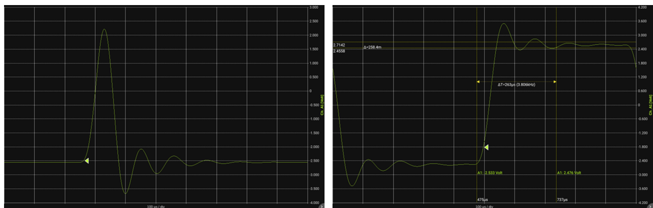
FIGURE 5.10 : Filtre passe-bas Chebyshev : Réponses impulsionnelle et indicielle
