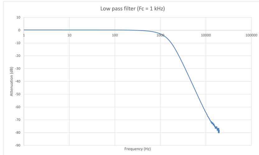
FIGURE 5.11 : Filtre passe-bas Bessel : Diagramme de Bode
