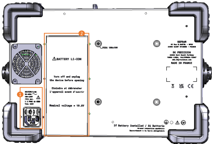
FIGURE 2.3 : Interfaces vue arrière
