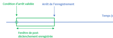
FIGURE 3.32 : Post-déclenchement
