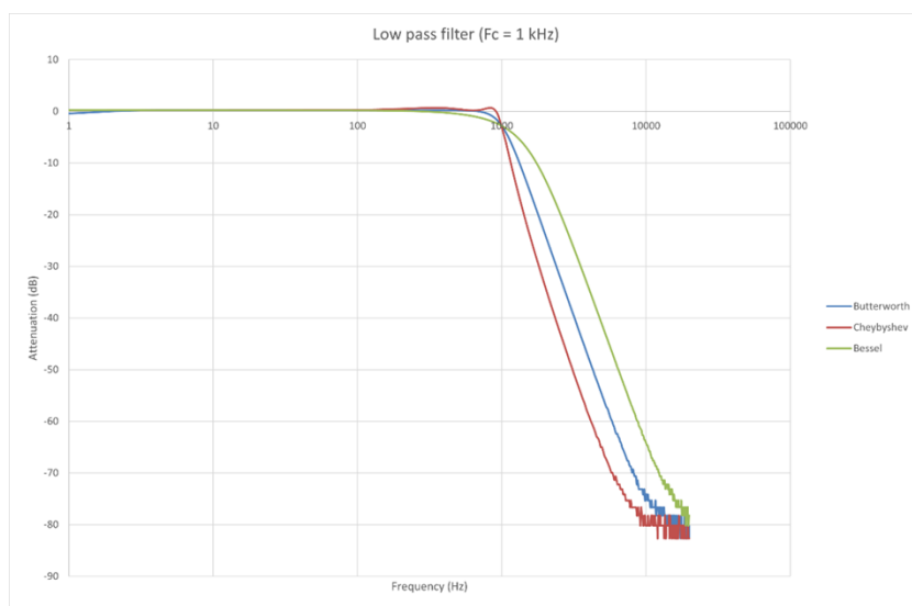
FIGURE 5.13 : Comparaison des filtres : Diagramme de Bode
