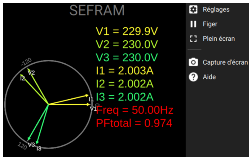
FIGURE 6.8 : Widget Diagramme de Fresnel
