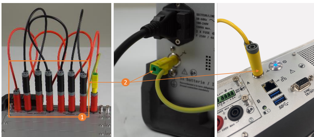
Figure 9.5: Raccordement des entrées universelles
