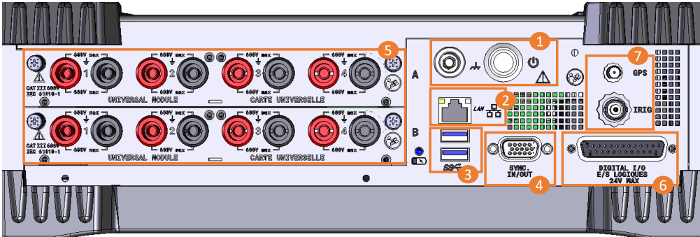
FIGURE 2.2 : Vue face de dessus
