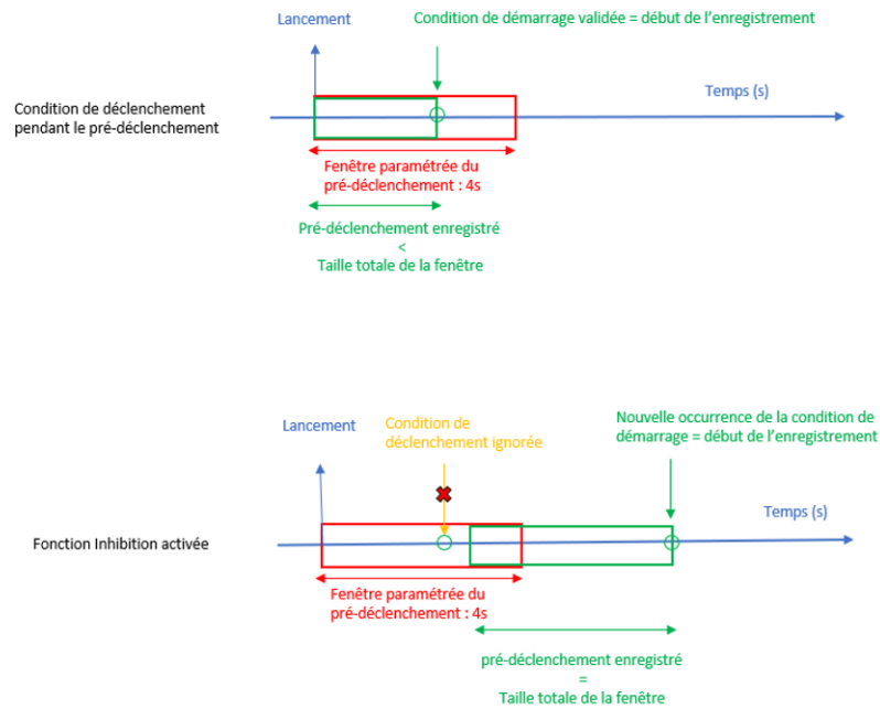
FIGURE 3.31 : Fonction inhibition
