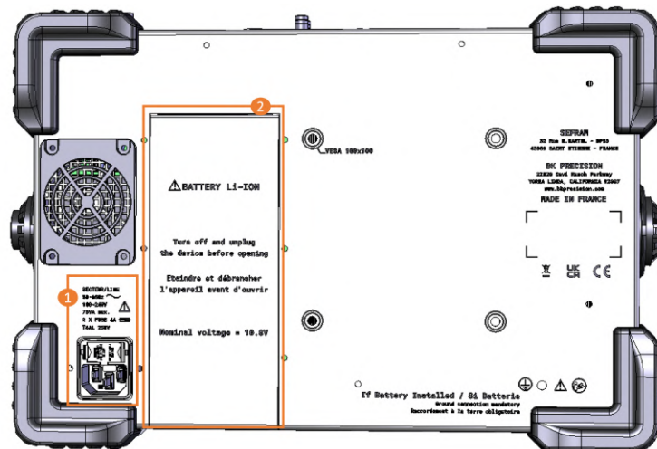
FIGURE 2.3 : Interfaces vue arrière
