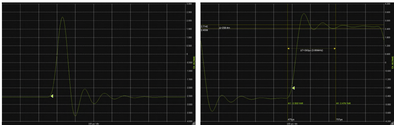
FIGURE 5.11 : Filtre passe-bas Chebyshev : Réponses impulsionnelle et indicielle
