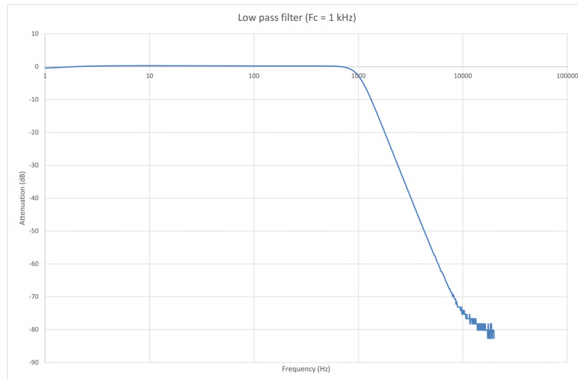
FIGURE 5.8 : Filtre passe-bas Butterworth : Diagramme de Bode
