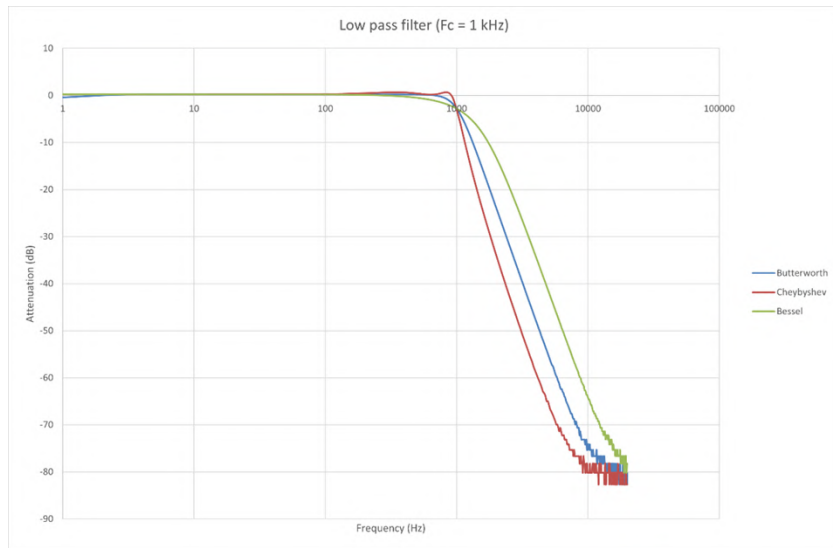
FIGURE 5.14 : Comparaison des filtres : Diagramme de Bode
