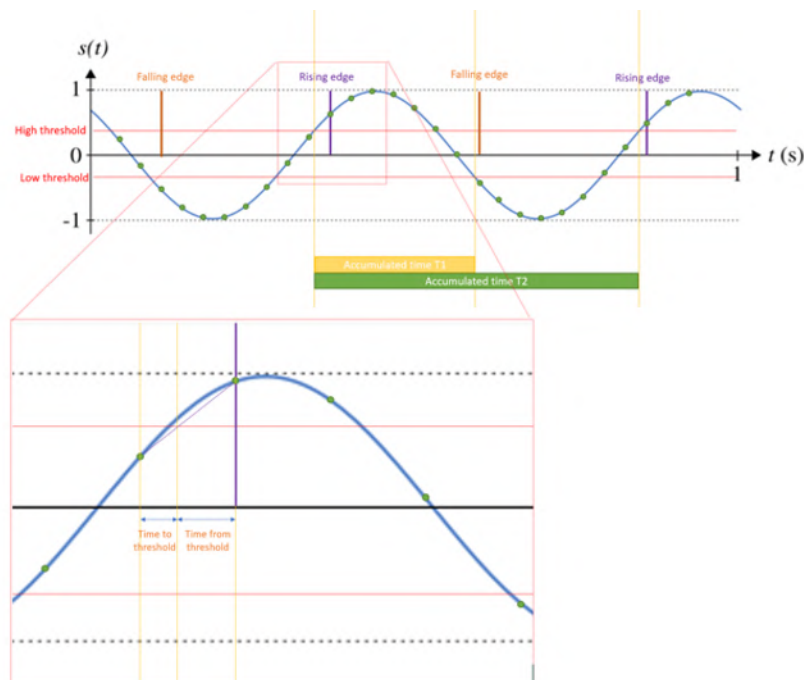
FIGURE 3.11 : Fréquence/PWM
