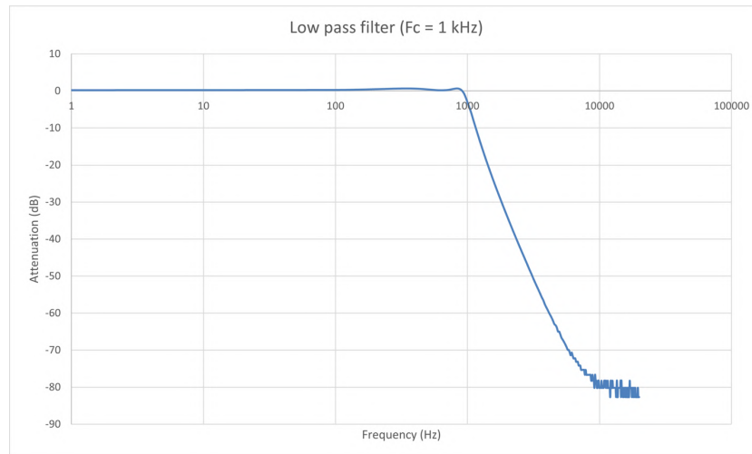
FIGURE 5.10 : Filtre passe-bas Chebyshev : Diagramme de Bode
