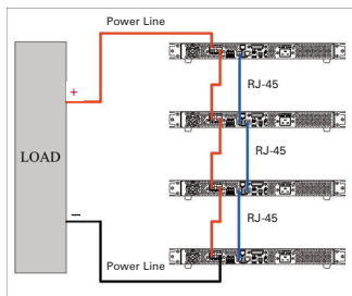
Configuración en Serie (Sólo en modelos de alta corriente)
