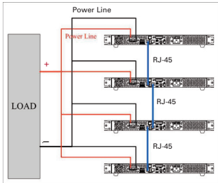
Configuración en Paralelo
