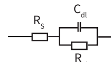
Células Randles simplificadas
