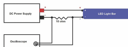
Ejemplo de configuración de prueba LED
