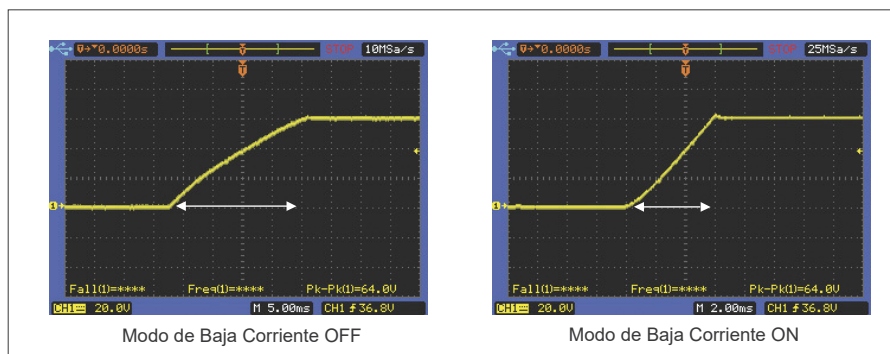
Tiempo de subida del voltaje con y sin el Modo de Baja Corriente habilitado
